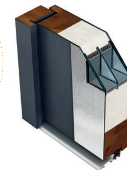
PRZEKRÓJ SKIRZYDŁA Z OŚCIEŻNICĄ ENERGO
