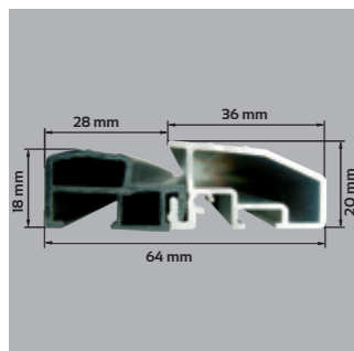
PRÓG ALUMINIOWY Z WIKŁADKĄ TERMICZNĄ
