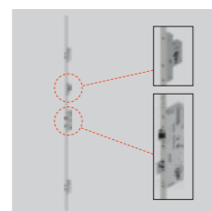
ZAMEK LISTWOWY Z DODATKOWYM GÓRNYM ZAMKIEM Z REGULOWANYMI ZACZEPAMI W OŚCIEŻNICY
